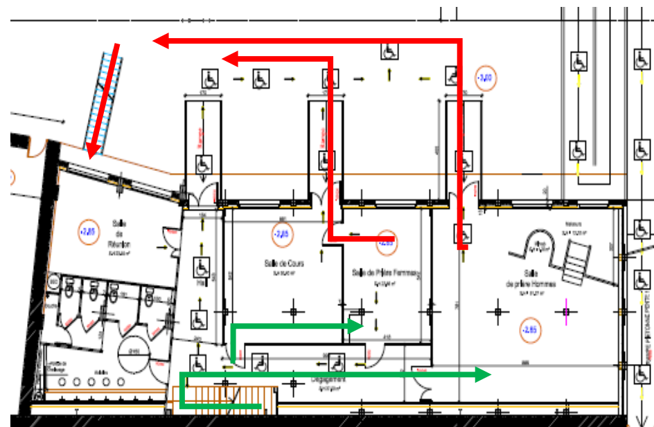
PLAN SOUS-SOL
